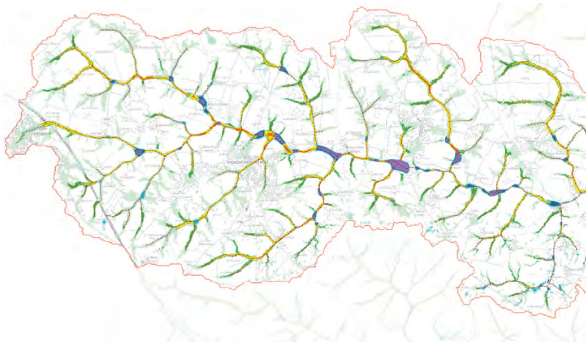
Fonctionnement hydraulique d'occurrence centennale - Le Gesvres
